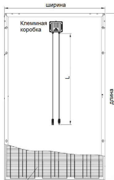
Вид спереди Рисунок 1 – схематическое изображение ФЭМ
